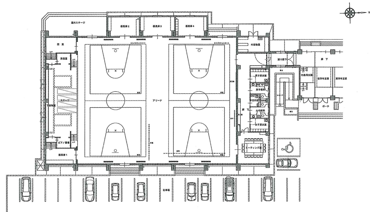
屋内運動場平面図
